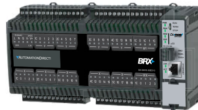
BRX 36E 36 Discrete I/O 6 Analog I/O Ethernet Port
